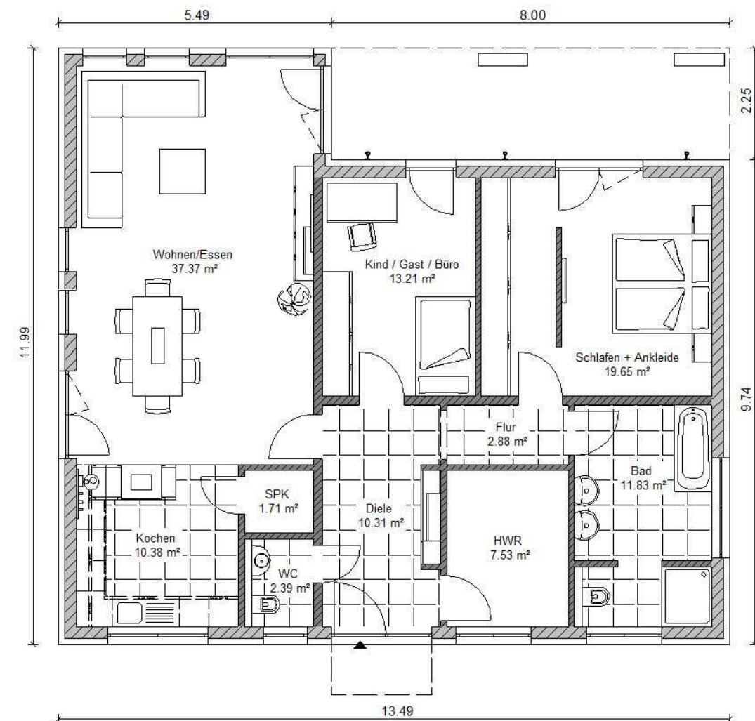
Grundriss
